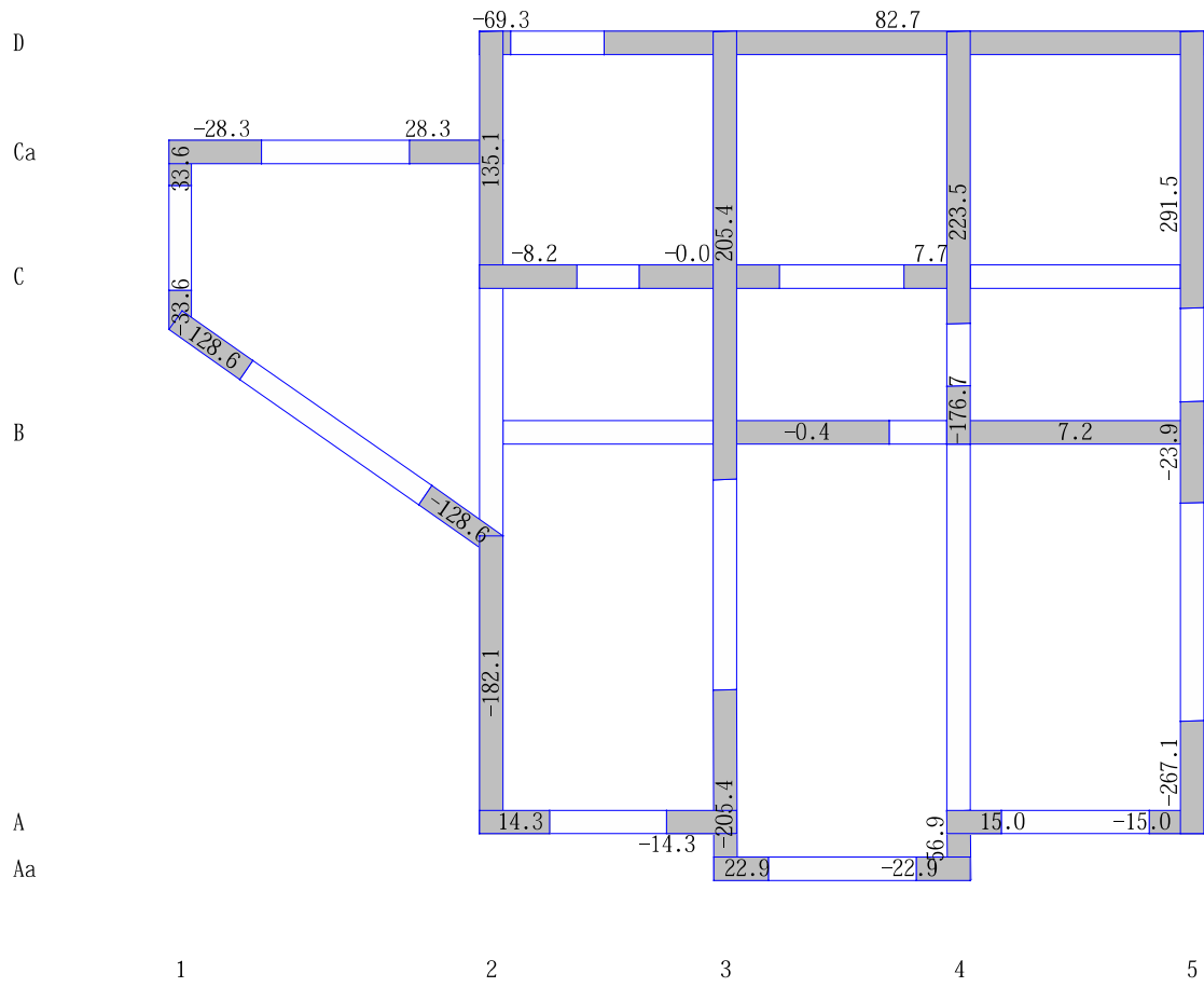
地震荷重時基礎反力図(Y加力) スケール:1/100
