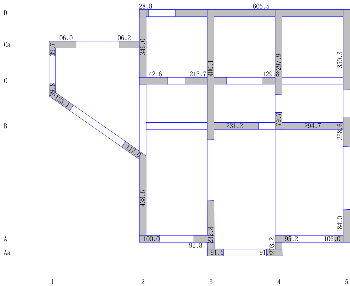
鉛直荷重時基礎反力図(合計=5436.2) スケール:1/100
